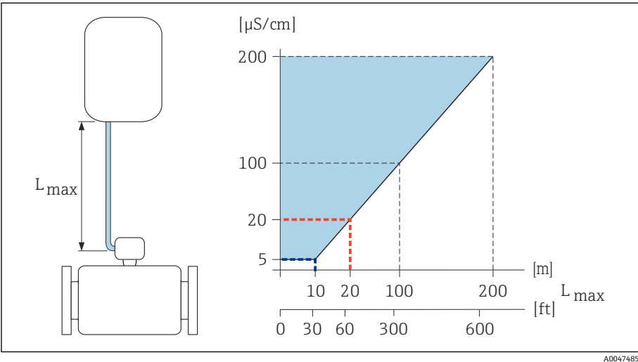
图 4 允许连接电缆长度
