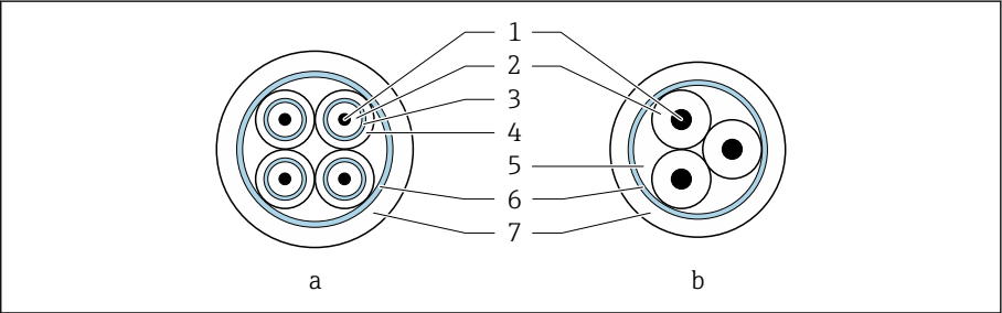
3 电缆横截面
